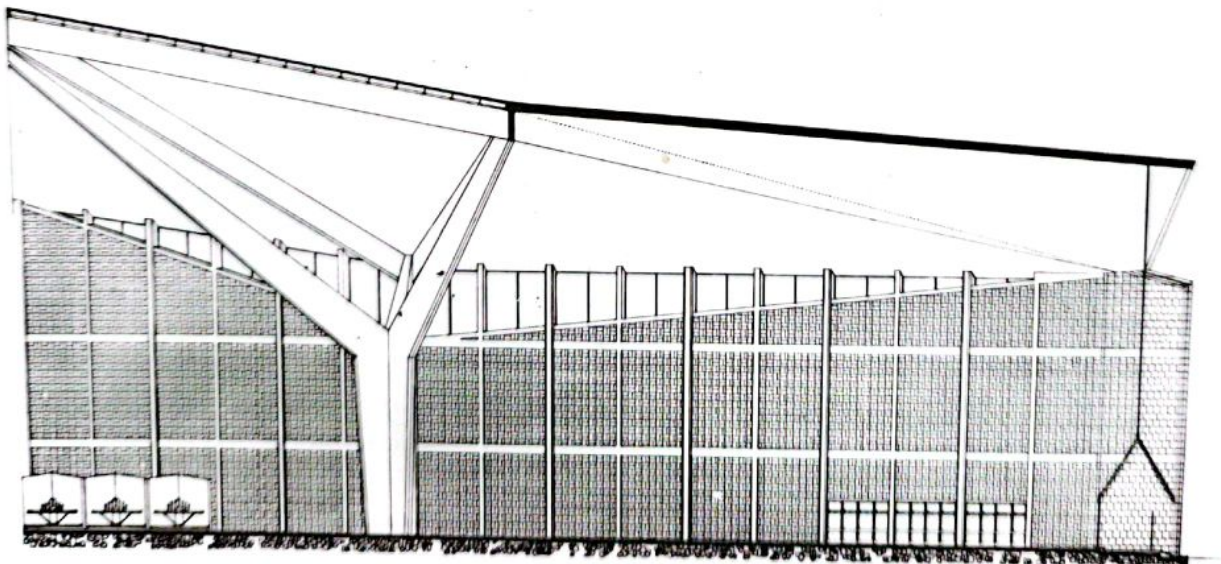
§ SEZIONE 1:100
