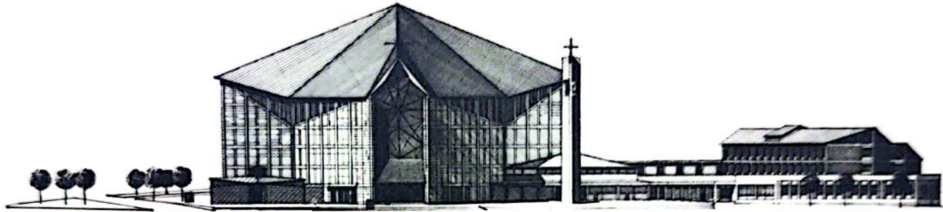
PROSPETTO 1:200
