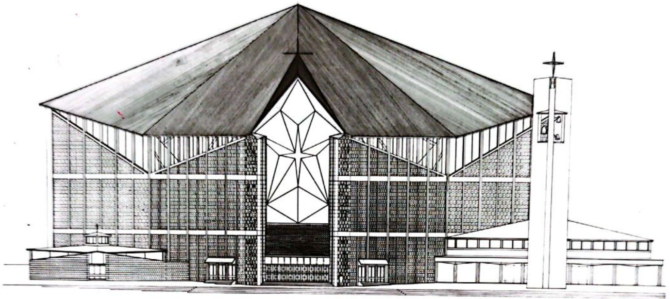
FACCIATA PRINCIPALE
