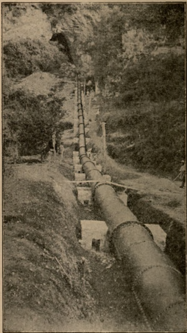
Fig. VI — Conduzione forzata di acciaio, che porta l'acqua dall'imboccatura della Grotta all'officina trasformatrice.
